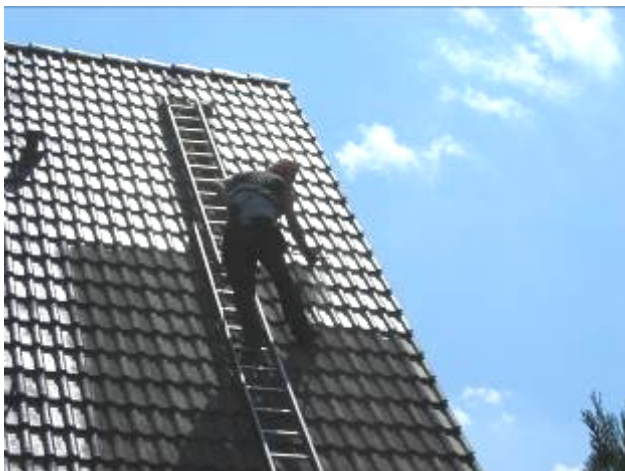
Grundierung und Endbeschichtung der Dachfläche in zwei Arbeitsgängen Auftrag der Grundierung
